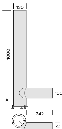
TUYAU VERTICAL (à commander en fonction du poêle à granulés souhaité)
